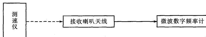
图 1 微波发射频率检定框图
