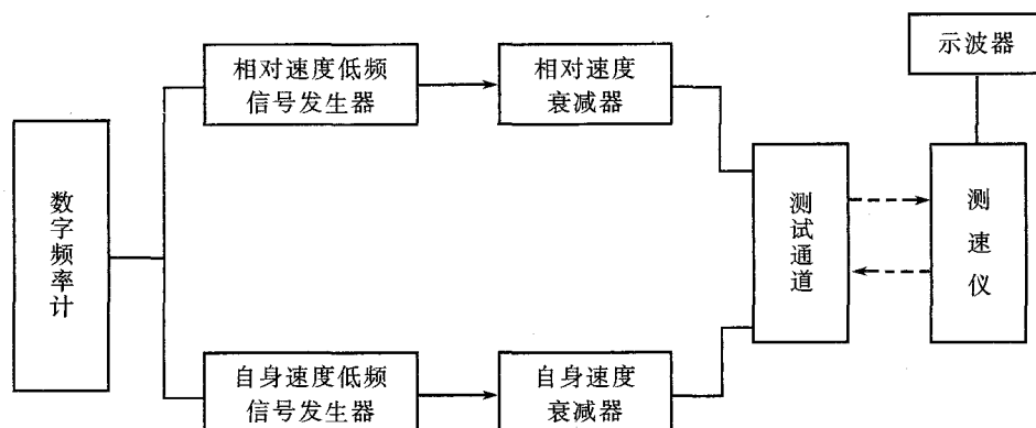
图 2 测速误差检定系统框图
